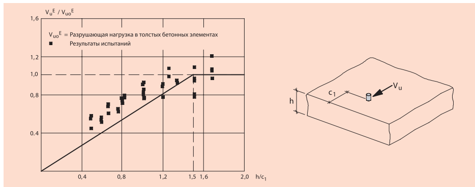
Рисунок 2.21: Влияние толщины основания h на несущую способность стальных анкеров, установленных вблизи края, при воздействии на них поперечной нагрузки
