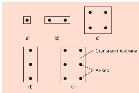
Рисунок 1а: Крепления на достаточном расстоянии от краев детали (любое краевое расстояние \geq 10 h_{ef} ) в соответствии с СС-Методом.
