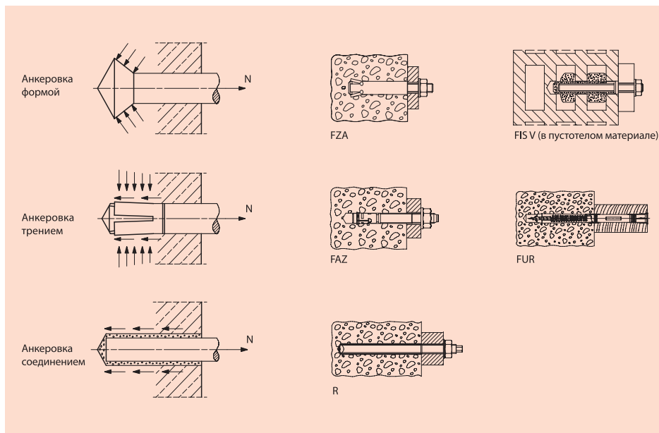
Рисунок 2.6: Принципы работы
