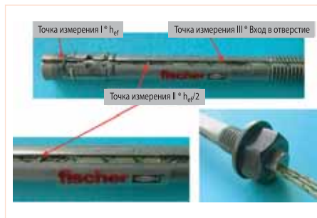
Рисунок 6.6: Измерение температуры анкерного болта FAZ в зависимости от расстояния до поверхности бетона
