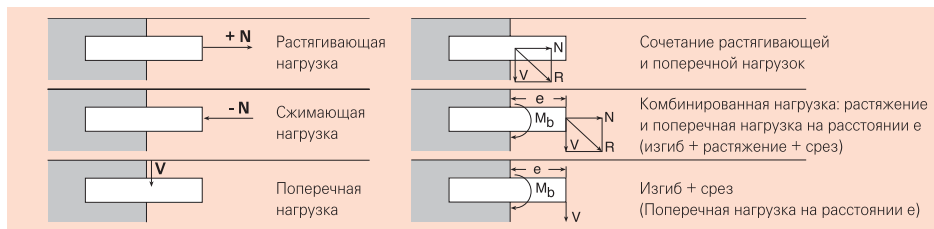
Рисунок 2.6: Принципы работы
