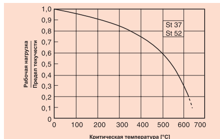
Рисунок 6.9: Характеристики стали в зависимости от температуры, взята из работы /9/
