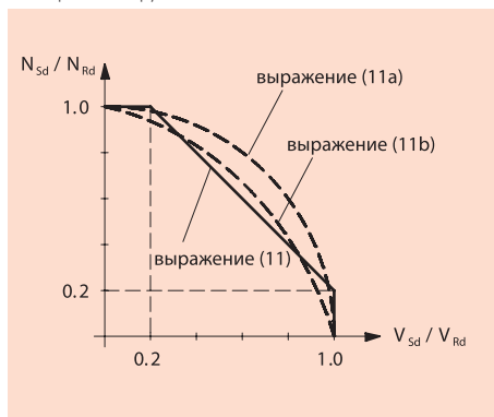
Рисунок 12: Схема взаимодействия комбинированной тяговой и поперечной нагрузки
