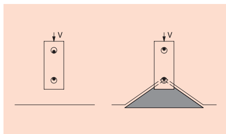
Рисунок 8: Типичное разрушение края бетонного элемента, происходящее в связи с неблагоприятной нагрузкой на анкера, установленные с гарантированным зазором (примечание: диаметры отверстий с гарантированным зазором преувеличены).
