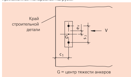
Рисунок 6: Пример крепления, находящегося под действием эксцентрично приложенной попересной нагрузки
