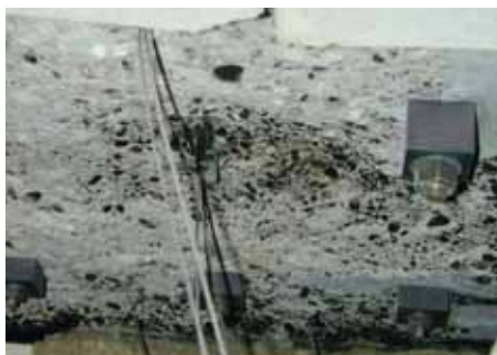
Рисунок 6.10: Откалывание поверхностного бетонного слоя /2/
