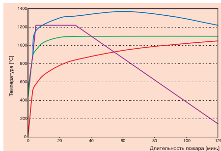
Рисунок 6.5: Кривые «температура/время» [7] — (ЕТК), — «углеродная» кривая, — «туннельная» кривая RABT Tunnel, — «туннельная» кривая Rijkswaterstaat Tunnel
