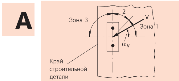
Рисунок 7: Определение угла \alpha_V
