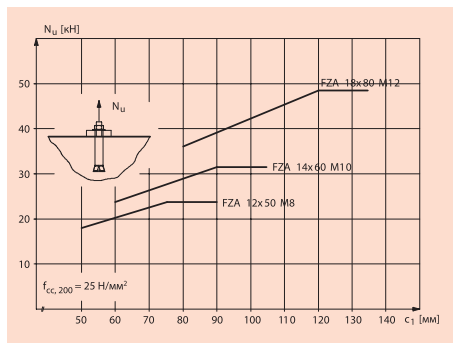
Рисунок 2.14: Предельные тяговые нагрузки N_U для анкера fischer Zykon (с выступающей резьбой) в неразрунутом бетоне в зависимости от краевого расстояния c_1 .
