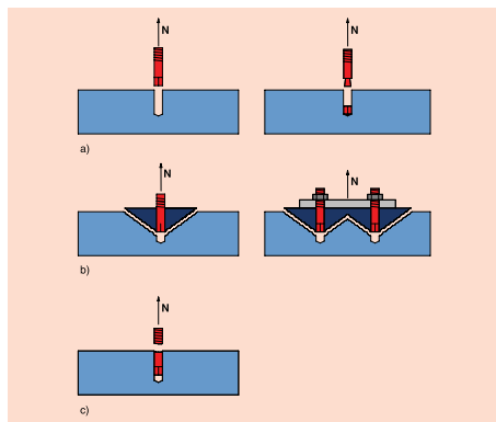
Рисунок 6.8: Типы разрушения под действием растягивающей нагрузки
