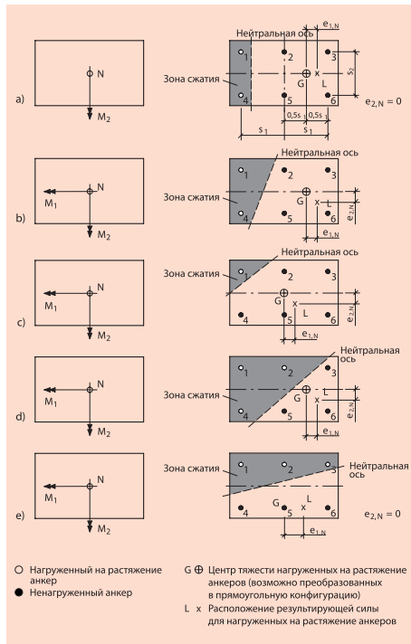
Рисунок 4: Примеры анкеров, испытывающих эксцентричные растягивающие нагрузки
