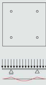
Крепеж посредством подрезных анкеров FZP
